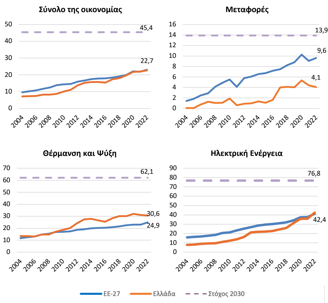
Διάγραμμα 2.4: Ποσοστό συμμετοχής ΑΠΕ στην κατανάλωση ενέργειας
