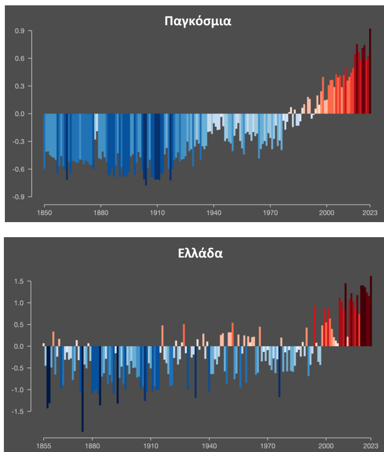
Διάγραμμα 2.1: Μεταβολή θερμοκρασίας ανά έτος, σε σχέση με την περίοδο 1961-2010, σε ^{\circ}\text{C}
